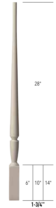
P2015 34" 38" 42"
