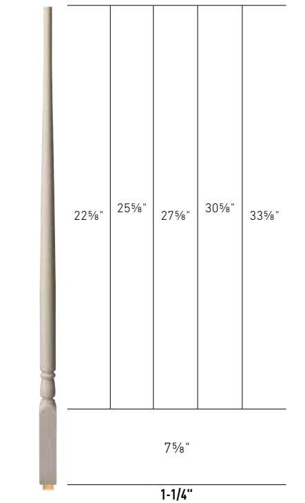
S 5015 31" 34" 36" 39" 42"
