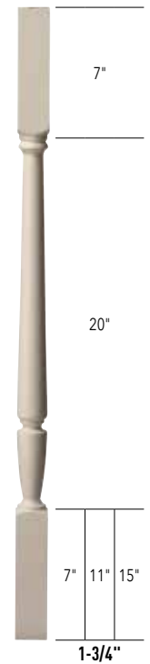
P2005 34" 38" 42"
